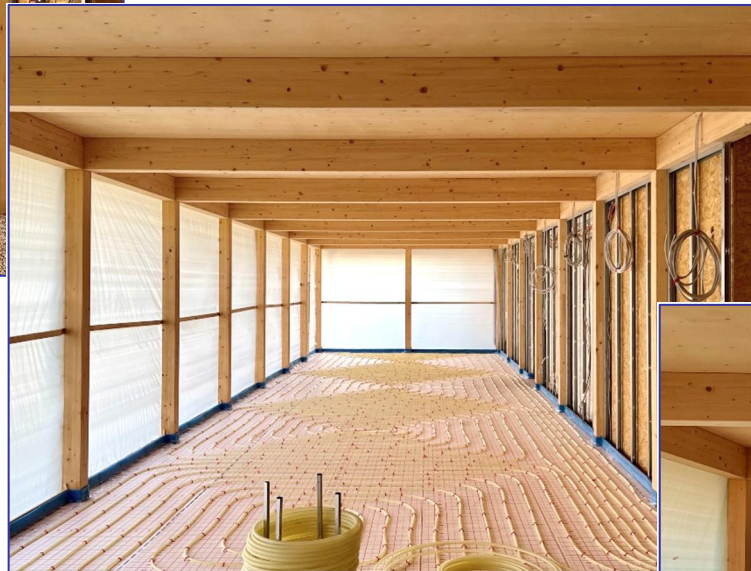
Schneckenförmig gelegte Polyethylen-Heizrohre
