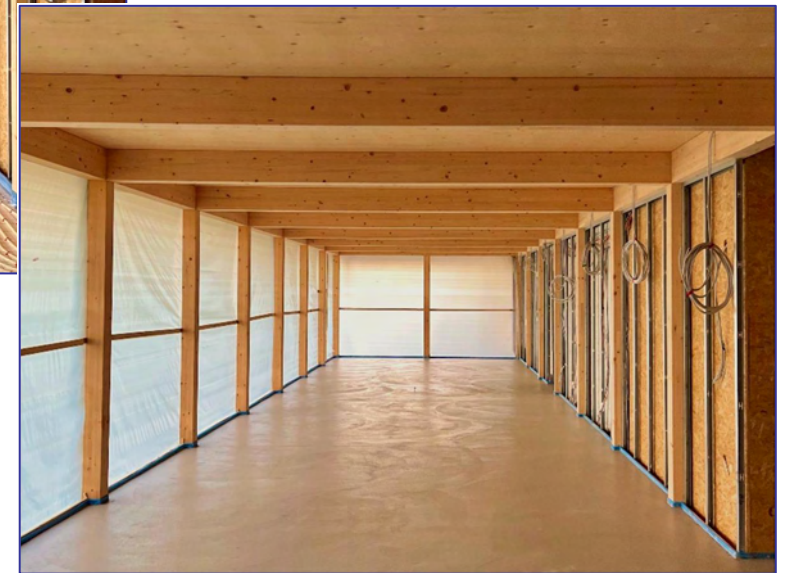
Schwimmender Fließestrich umschließt die Fußbodenheizung
